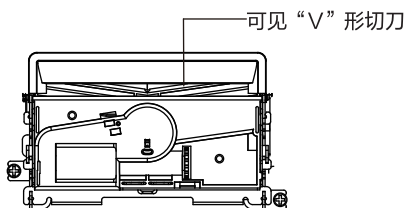
卡刀时，切刀未缩回，可见切刀 图（1）
